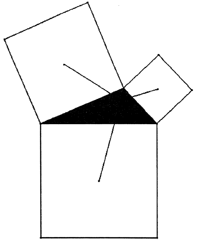
共點
