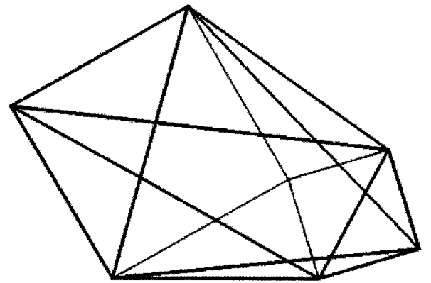
等面積
