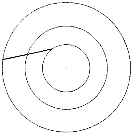
等長
