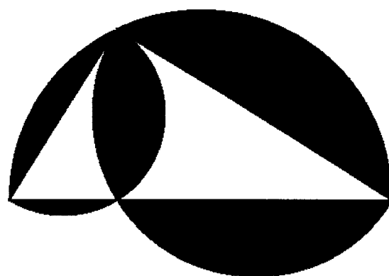
等面積
