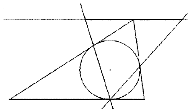
等長
