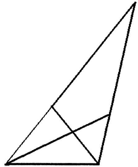
等比
