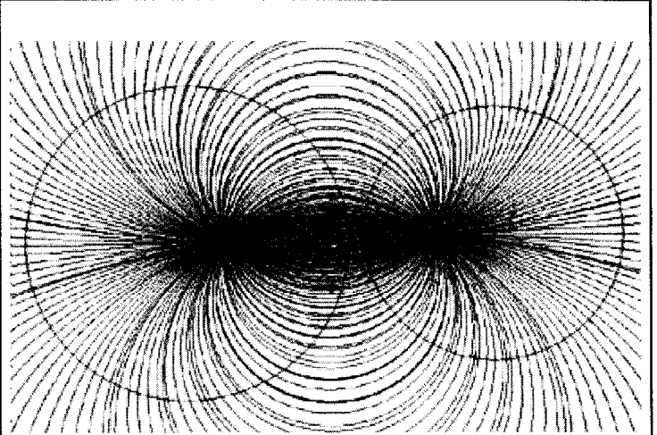
共軸圓束
