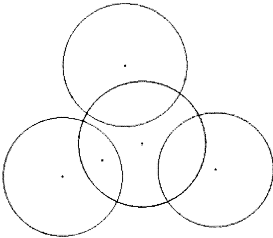
正交
