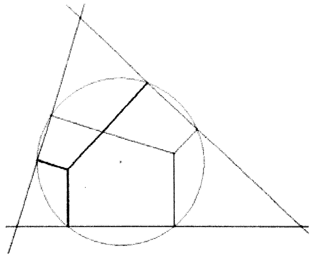
垂直・共點
