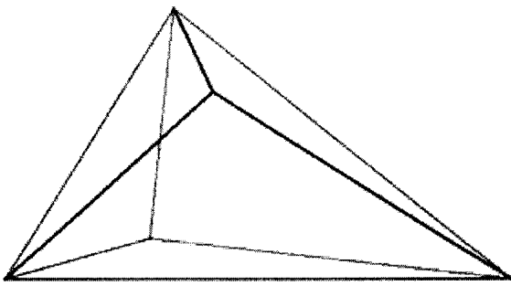
共點
