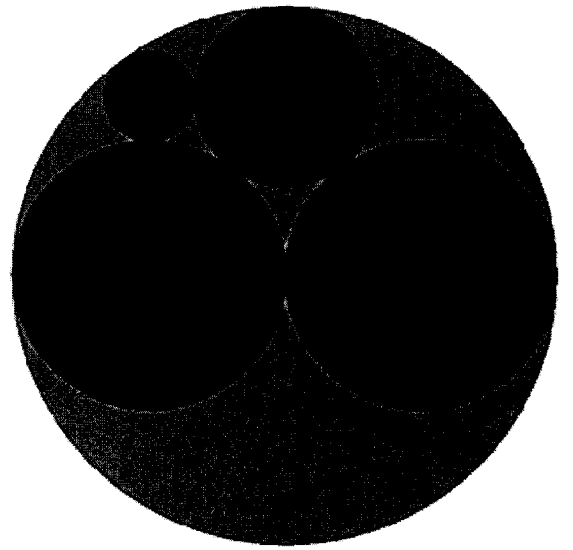
半徑關係
