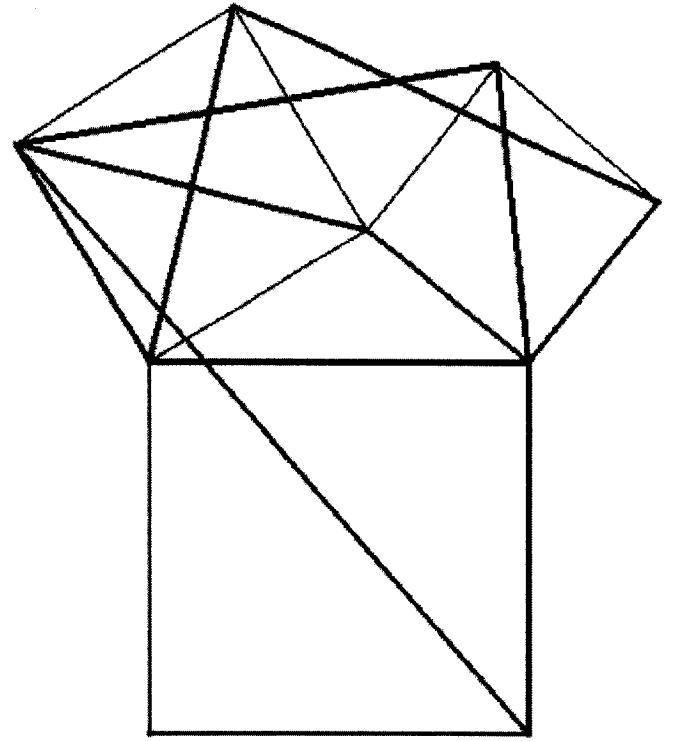
等面積
