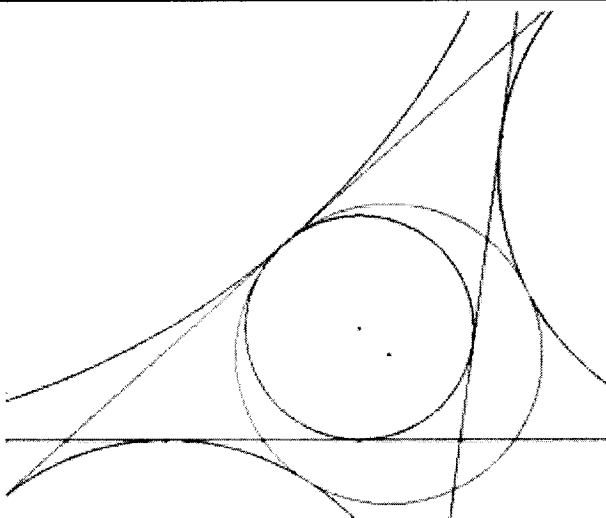
內切圓、傍切圓、九點圓
