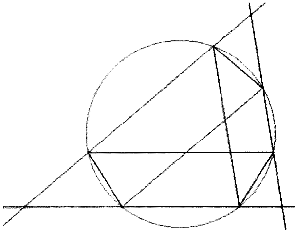
共圓
