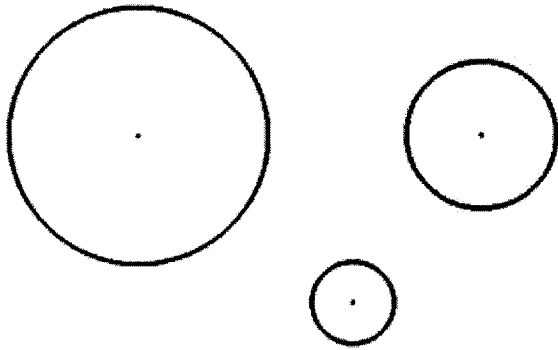
三個圓
