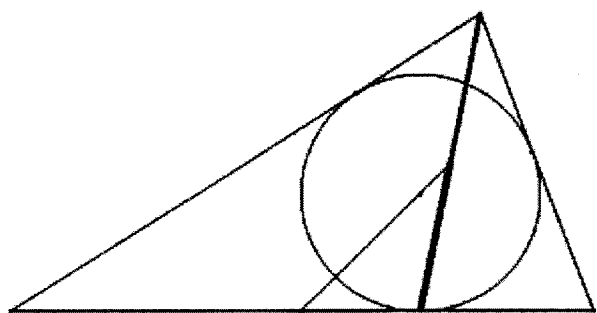
等長
