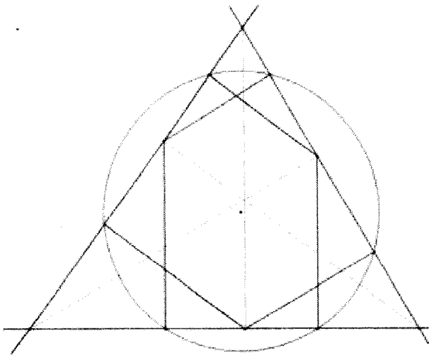
共圓
