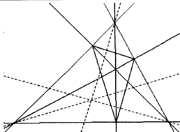
共點
