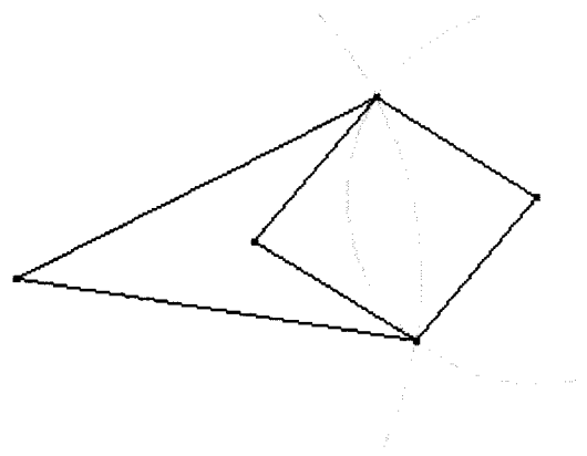
連動桿
