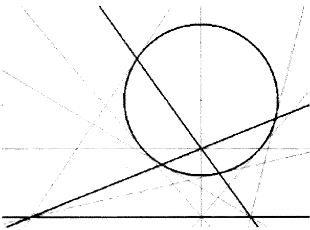
自配極三角形
