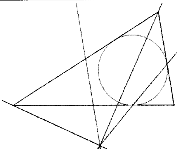
共點
