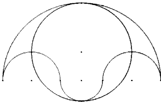
等面積
