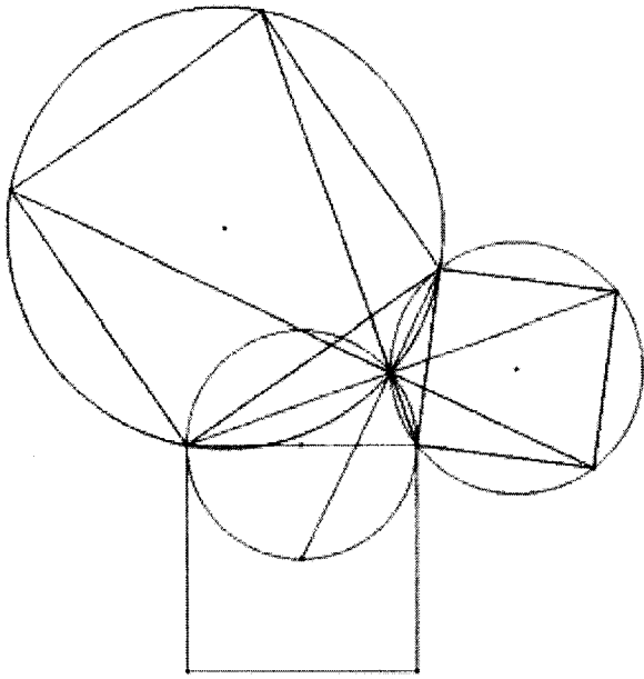
共點
