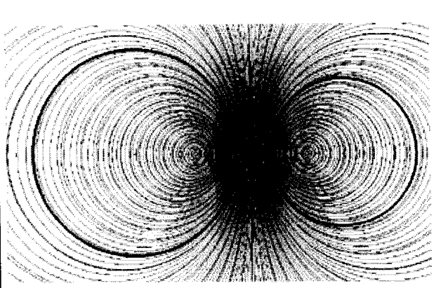
共軸圓束
