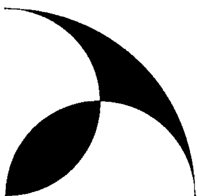
等面積
