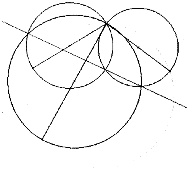
共線
