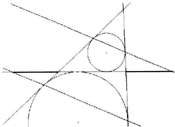
等長
