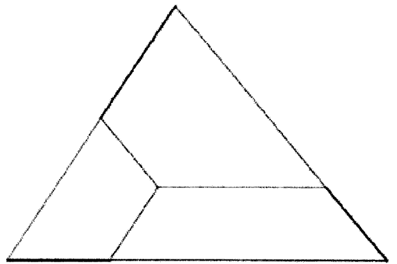
比例和 = 1
