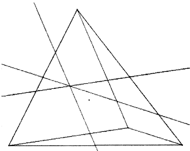
共點
