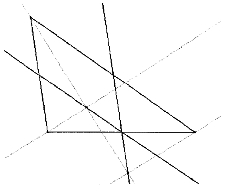
共點
