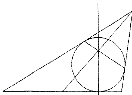
共點
