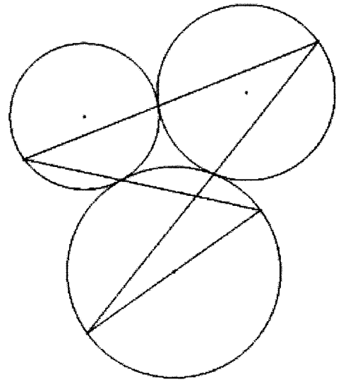
回到對面
