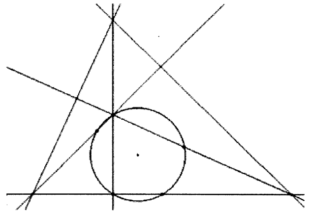
共圓
