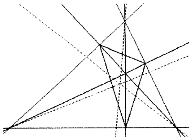
共點
