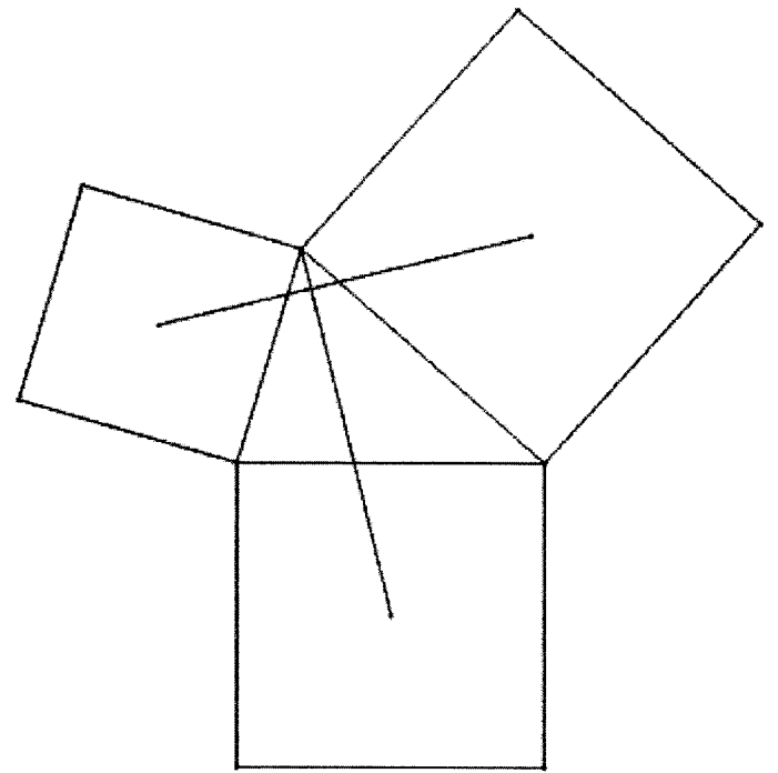
等長 垂直
