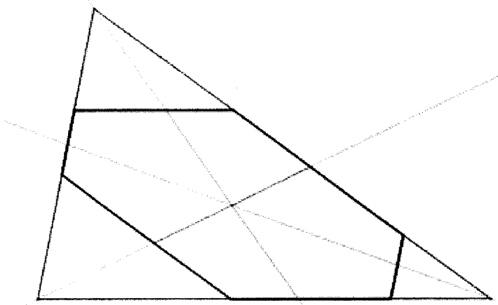
等長
