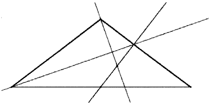
垂直
