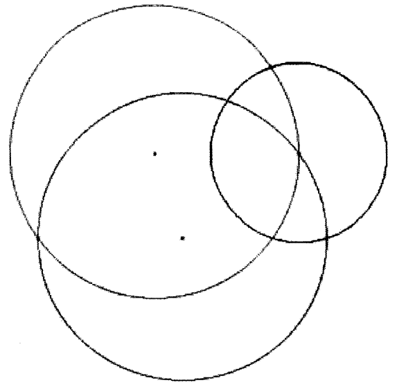
共線
