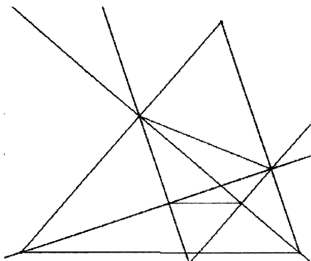
等比
