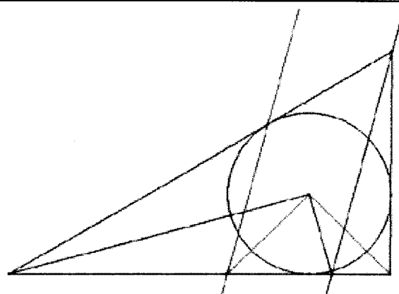
平行
