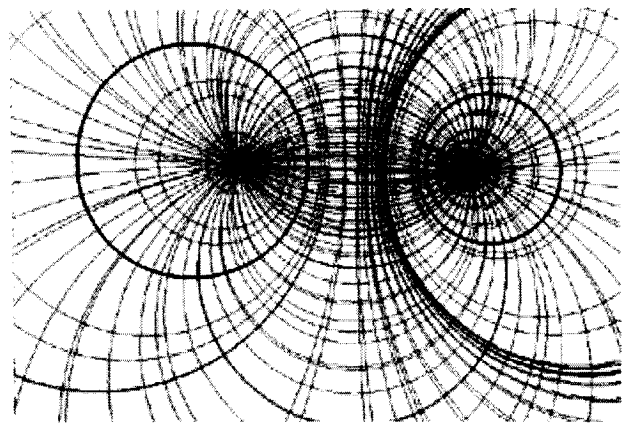
正交共軸圓束
